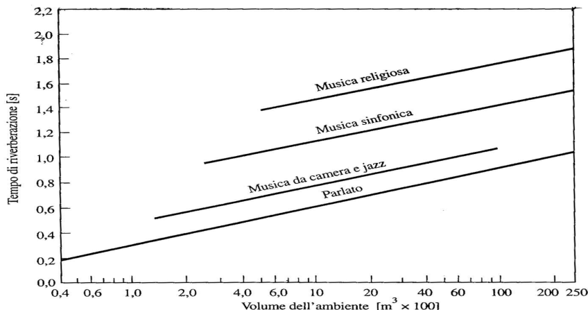
Tempi di riverberazione ottimale (500 Hz)
